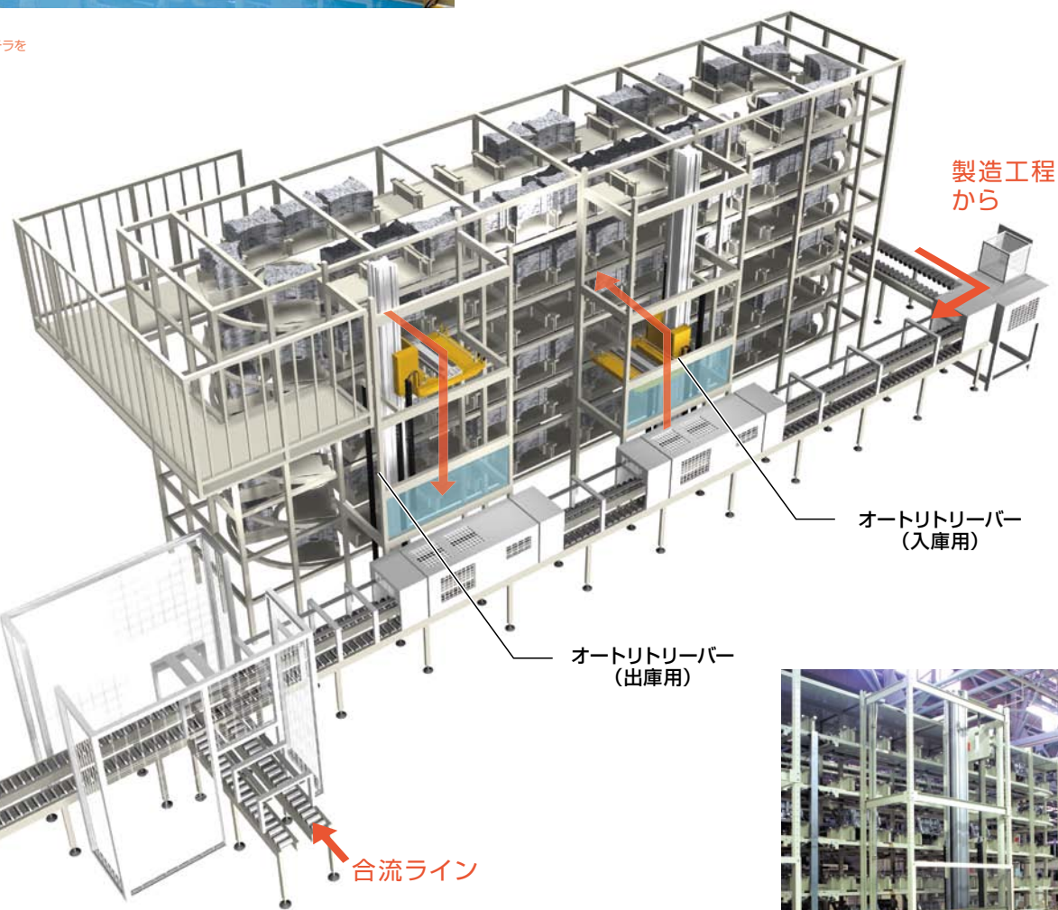
多段式独立水平回転棚
