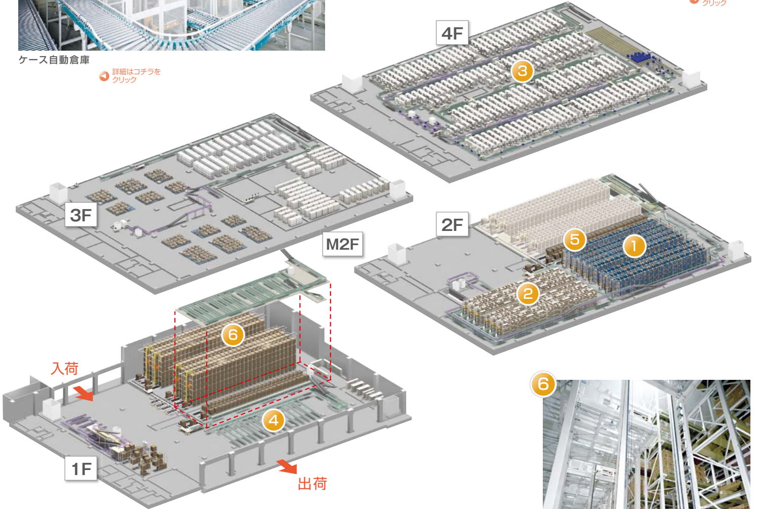
ボックス品ピッキングエリア
